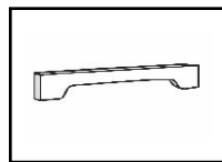
VA_24 3 1/2"H X 24"L X 3/4"TH VA_30 3 1/2"H X 30"L X 3/4"TH VA_36 3 1/2"H X 36"L X 3/4"TH VA_42 3 1/2"H X 42"L X 3/4"TH VA_48 3 1/2"H X 48"L X 3/4"TH
