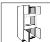
OV_24 24"W X 84"H X 24"D OV_27 27"W X 84"H X 24"D OV_30 30"W X 84"H X 24"D
